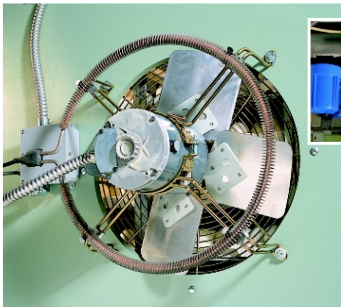
ELEMENTO TÉRMICO EN FORMA DE ANILLO MONTADO EN LOS VENTILADORES
